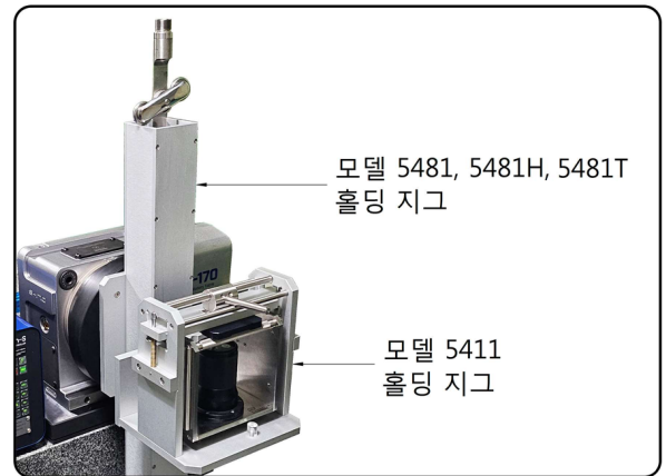
[홀딩 지그]
